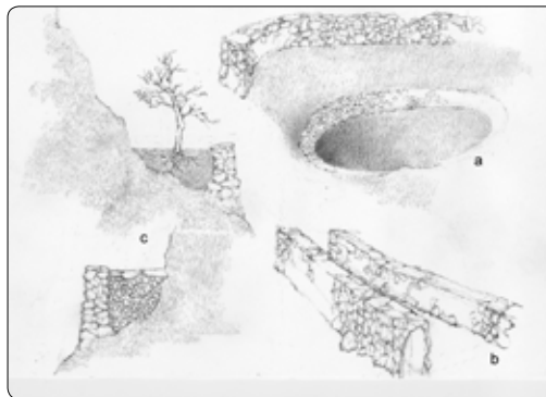
Kal, v poglobljenem reliefu, prilagojen prostor za zbiranje in rabo vode; b) S suhim zidom opredeljena pot, ki organizira gibanje v naselju in zagotavlja dostopnost na območju; c) Suhi zid kot zaščita humusa in opora pohodni površini. Risba: Josip Korošec, 2015.
